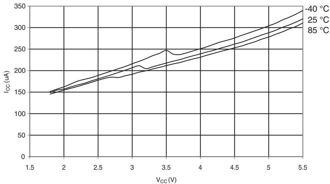
Figure 31-324. ATmega328: ADC Current vs. V CC (AREF = AV CC )
